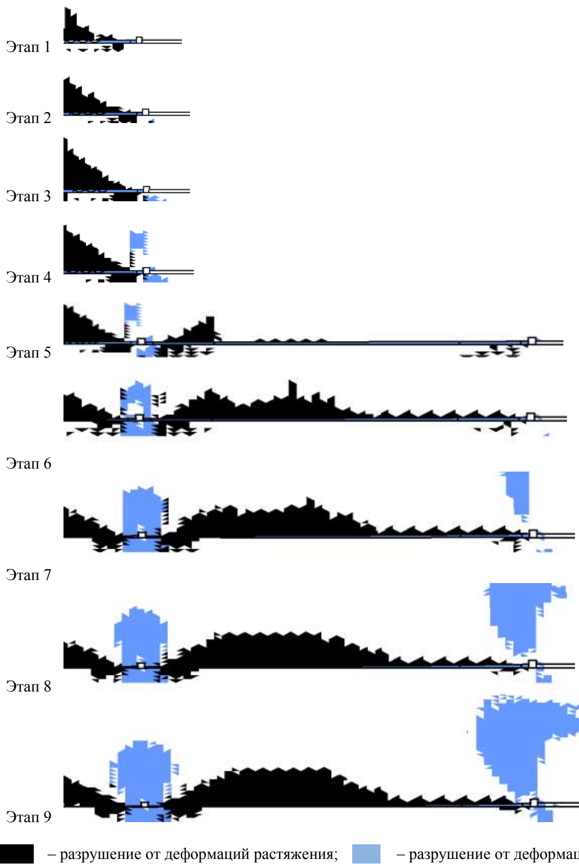
Рисунок 4 – Формирование зон разрушения при отработке смежных выемочных участков Следует отметить, что при отработке одной лавы, как и при отработке
