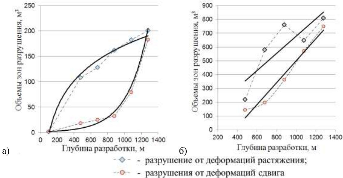
Рисунок 5 – Динамика развития зон разрушения в породах кровли смежных выемочных участков при отработке одиночной лавы (а) и дальнейшей отработке смежной лавы (б) с учетом характера деформаций геомеханической системы
