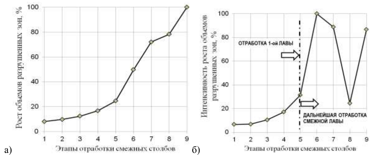
Рисунок 6 – Закономерности увеличения объемов (а) и интенсивности роста разрушенных зон в породном массиве при отработке смежных участков
